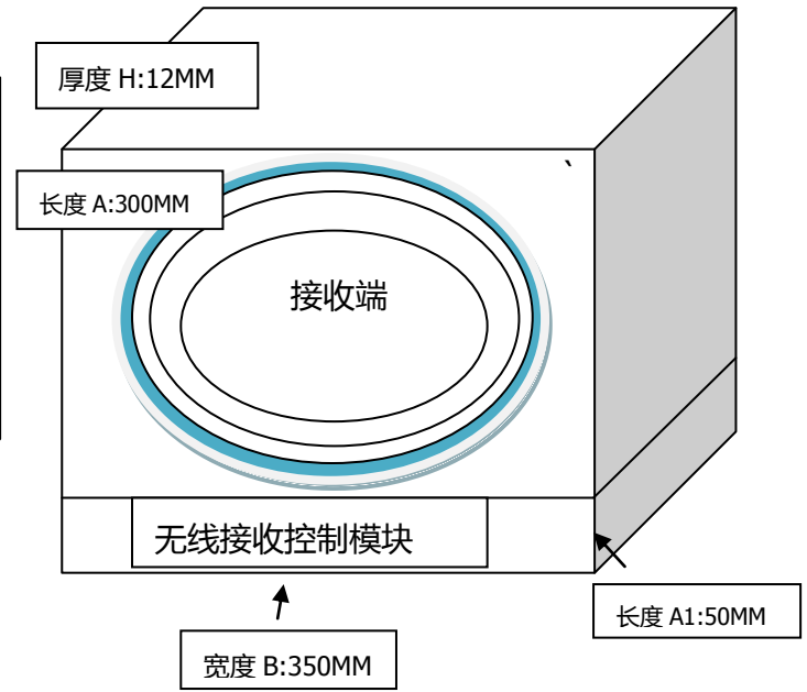
图四：接收线盘
