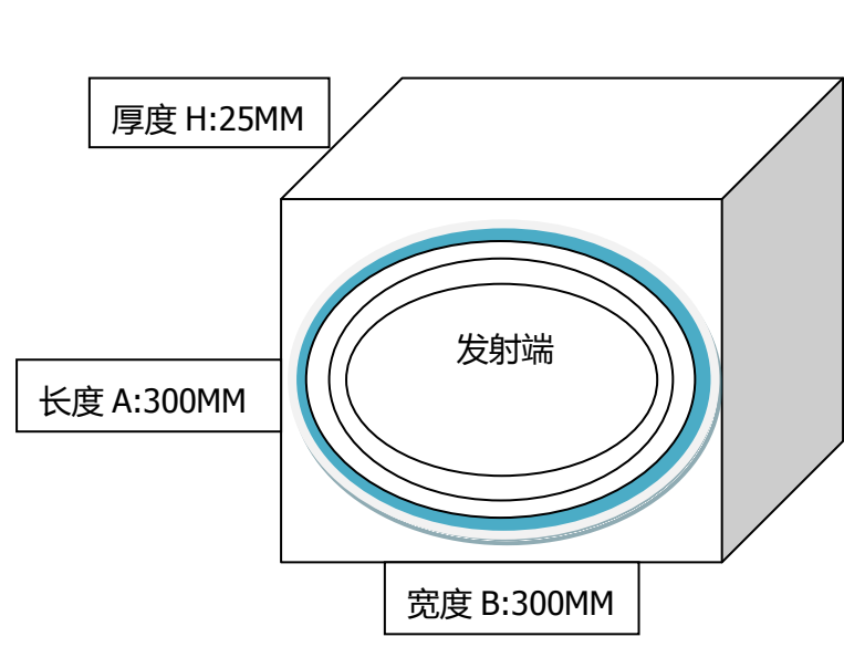
图三：发射箱体
